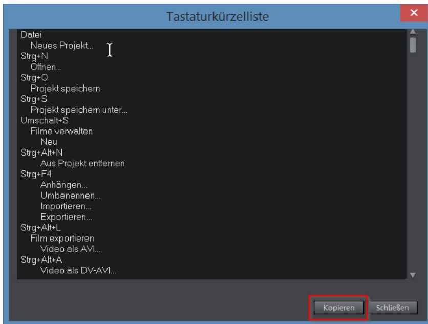
Abbildung 3: Tastaturkürzelliste
