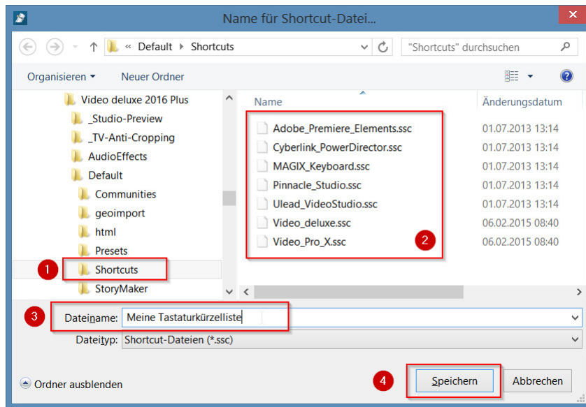
Abbildung 2: Tastaturkürzelliste speichern
